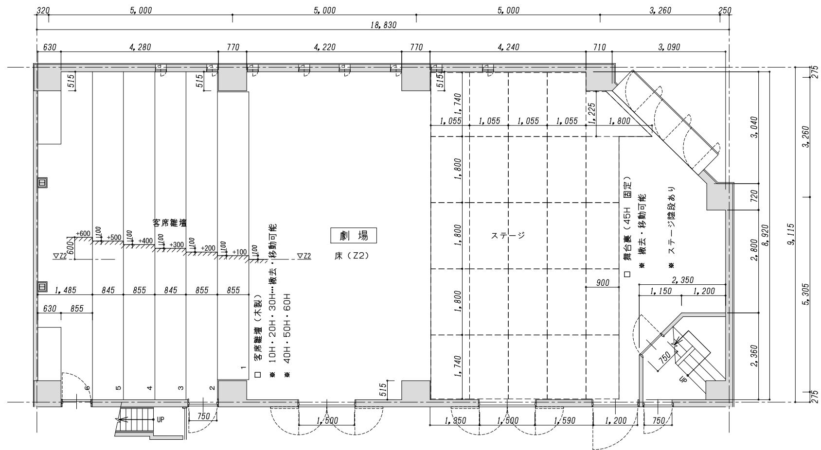
2階 平面図 1:100 (2階床 Z2)
