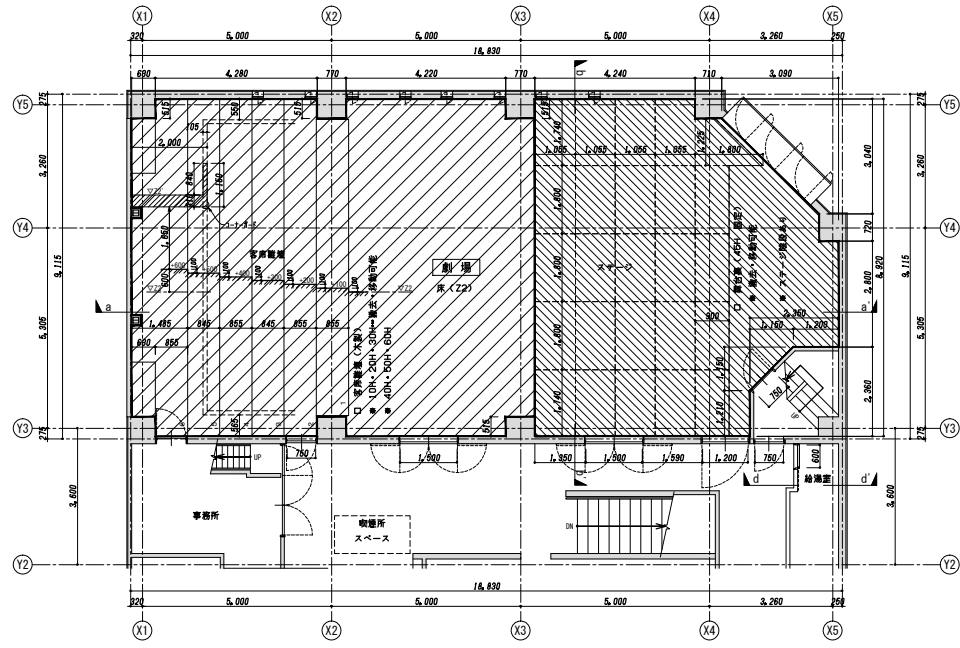
2階 平面図 (2階床 Z2)
