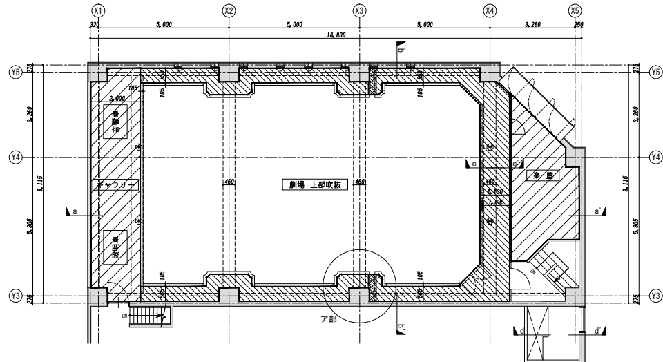
3階 平面図 (3階床 Z2')
